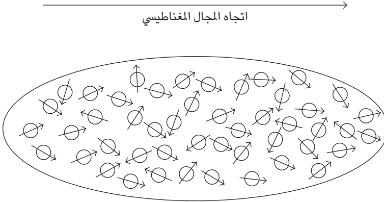
شكل ١-١: البارامغناطيسية.
